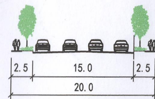
C-C 体育北路道路横断面
